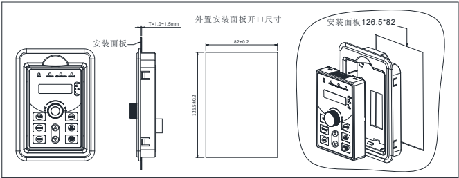
附：PI550A1/PI550A 键盘仓尺寸图(尺寸单位：mm)：
